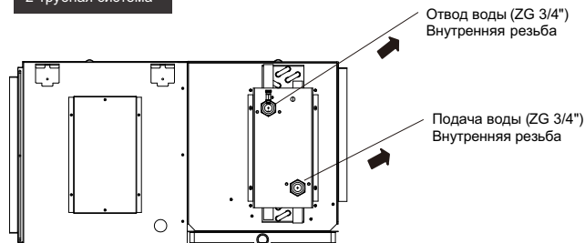
2-трубная система
